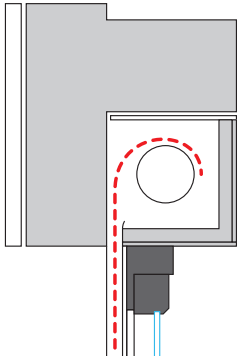
Enroulement intérieur derrière linteau
