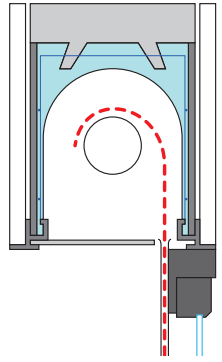
Enroulement extérieur dans coffre linteau
