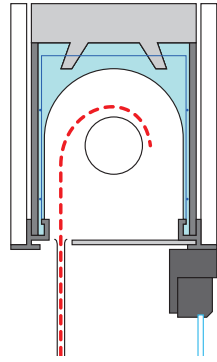
Enroulement intérieur dans coffre linteau
